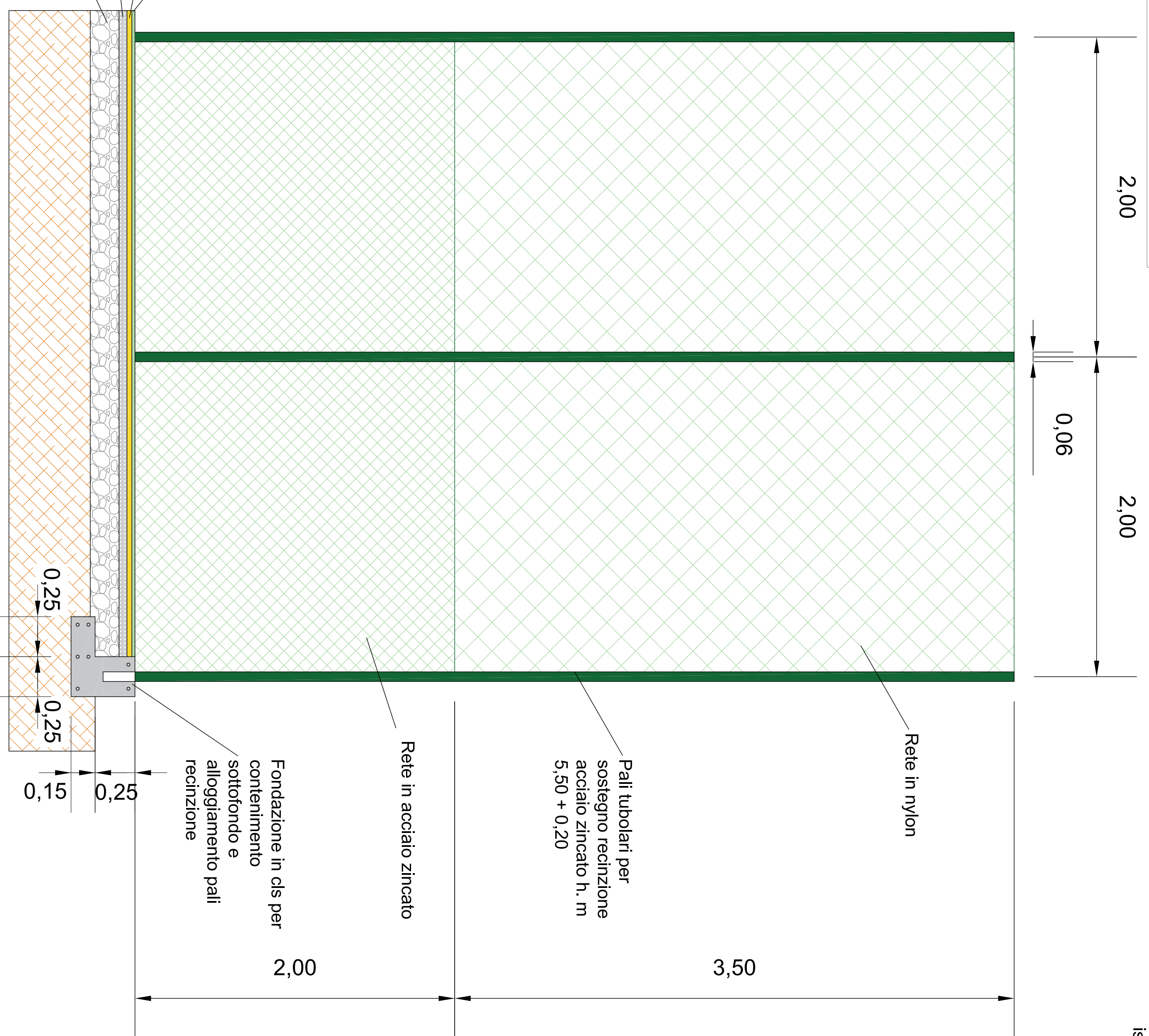
Sezione Tipo - Scala 1:20
