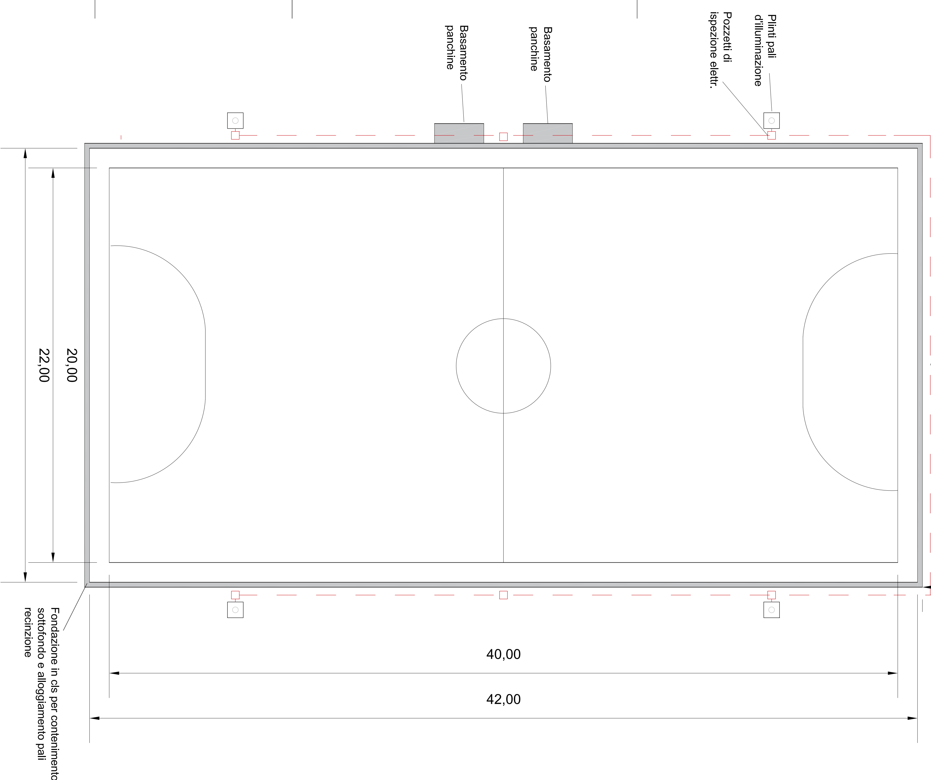
Pianta - Scala 1:100
